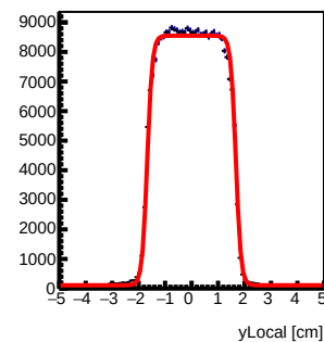
Tray100 : y Local Fit
