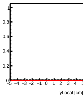
Tray118 : y Local Fit
