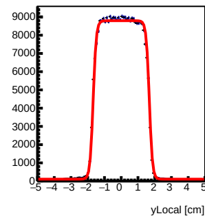
Tray84 : y Local Fit
