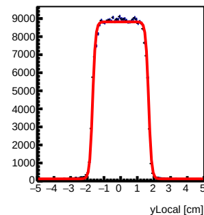
Tray92 : y Local Fit
