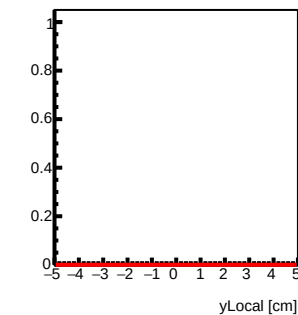
Tray88 : y Local Fit
