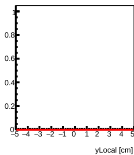
Tray101 : y Local Fit
