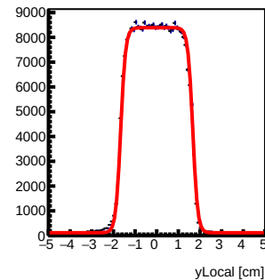
Tray96 : y Local Fit
