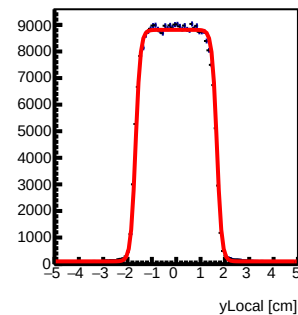
Tray24 : y Local Fit
