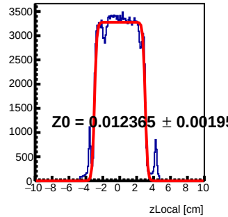
Module 6 Tray61 : z Local Fit
