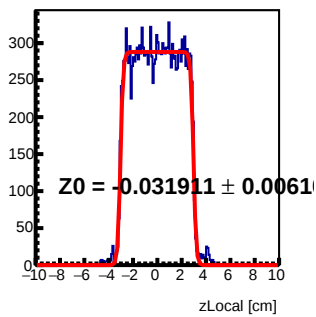
Module 2 Tray115 : z Local Fit
