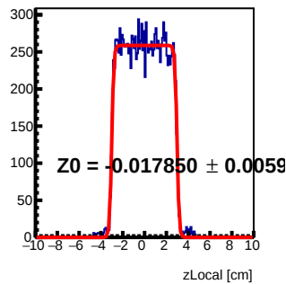
Module 2 Tray45 : z Local Fit
