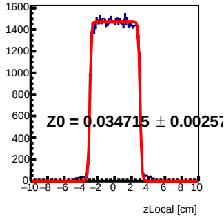
Module 3 Tray28 : z Local Fit
