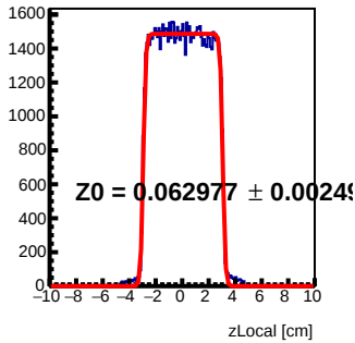
Module 3 Tray29 : z Local Fit
