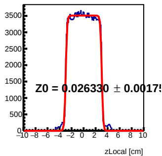
Module 6 Tray109 : z Local Fit
