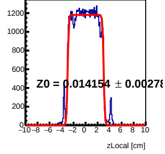
Module 4 Tray92 : z Local Fit
