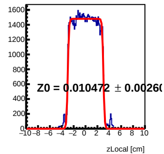
Module 3 Tray87 : z Local Fit
