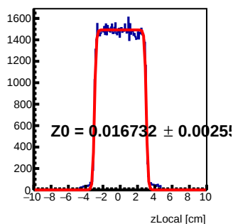
Module 3 Tray18 : z Local Fit
