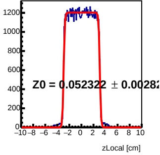
Module 4 Tray73 : z Local Fit
