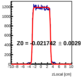
Module 4 Tray37 : z Local Fit
