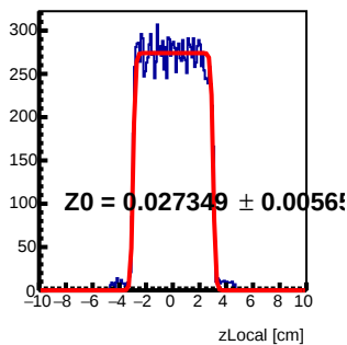
Module 2 Tray35 : z Local Fit
