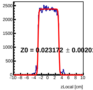
Module 6 Tray93 : z Local Fit
