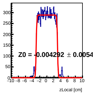
Module 2 Tray117 : z Local Fit
