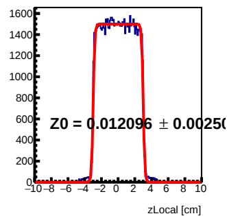
Module 3 Tray23 : z Local Fit
