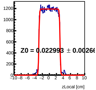
Module 4 Tray84 : z Local Fit
