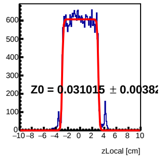
Module 1 Tray93 : z Local Fit
