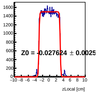
Module 3 Tray54 : z Local Fit
