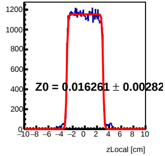
Module 4 Tray80 : z Local Fit
