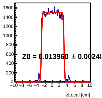
Module 3 Tray113 : z Local Fit
