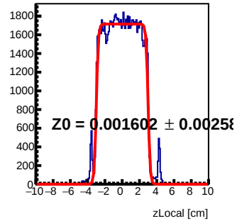
Module 0 Tray116 : z Local Fit
