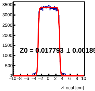
Module 6 Tray51 : z Local Fit
