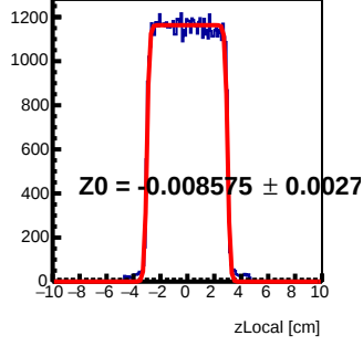
Module 4 Tray70 : z Local Fit
