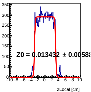
Module 2 Tray63 : z Local Fit
