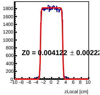
Module 0 Tray94 : z Local Fit
