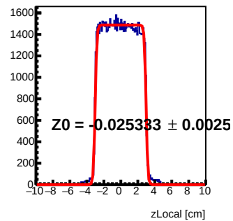
Module 3 Tray47 : z Local Fit
