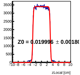
Module 6 Tray50 : z Local Fit
