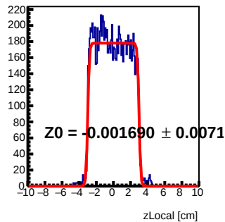
Module 2 Tray4 : z Local Fit
