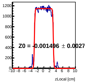
Module 4 Tray111 : z Local Fit
