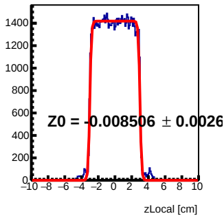
Module 3 Tray105 : z Local Fit
