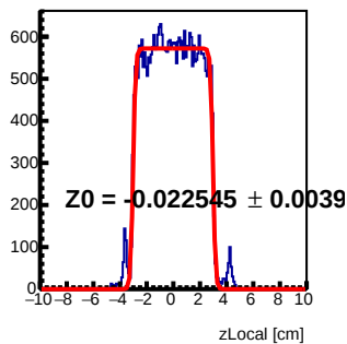
Module 1 Tray106 : z Local Fit
