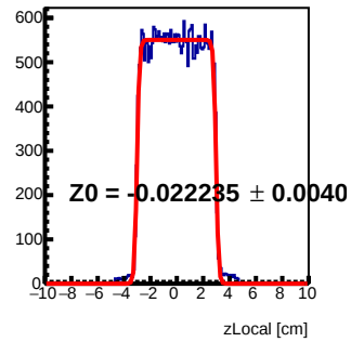
Module 1 Tray45 : z Local Fit
