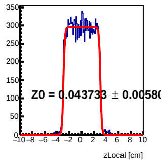
Module 2 Tray38 : z Local Fit
