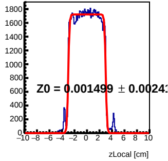
Module 0 Tray106 : z Local Fit
