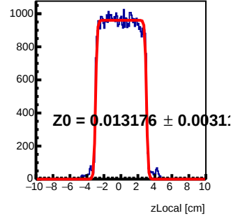
Module 4 Tray95 : z Local Fit
