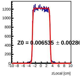
Module 4 Tray18 : z Local Fit
