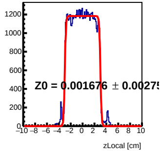
Module 4 Tray82 : z Local Fit
