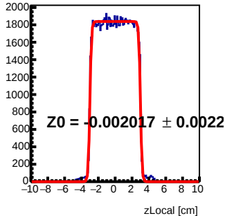
Module 0 Tray9 : z Local Fit
